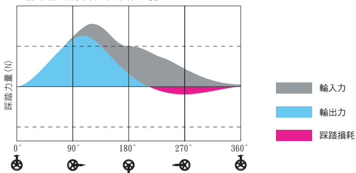
左腳踩踏力顯示圖(一次踩踏360度)
