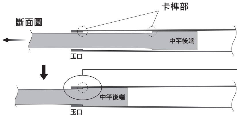
圖1卡榫固定著竿節的狀態。
